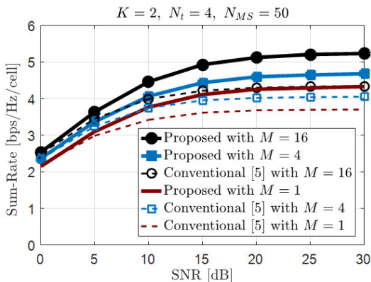
그림 1. SNR에 따른 제안한 기법의 데이터 전송률 성능 Fig. 1. Sum-rate performance of the proposed technique according to the input SNR.
