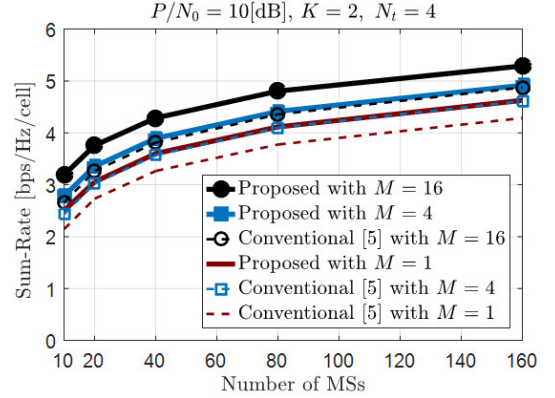
그림 2. 단말 수에 따른 제안한 기법의 데이터 전송률 Fig. 2. Sum-rate performance of the proposed technique according to the number of MSs in each cell.
